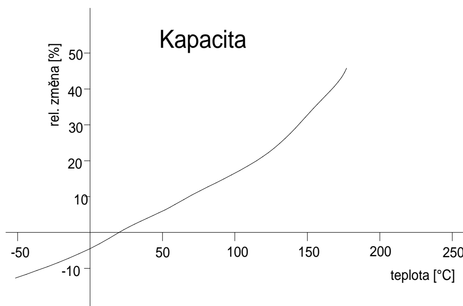
Obr. 4 Teplotní závislost kapacity snímačů
