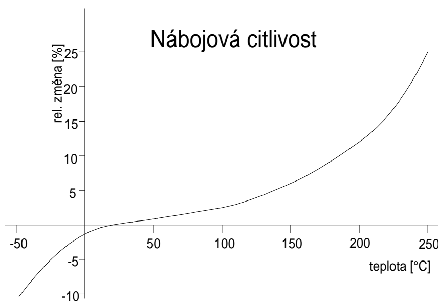
Obr. 3 Teplotní závislost nábojové citlivosti snímačů
